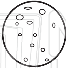
Venus
